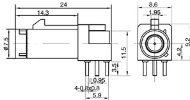
FAKRA SMB-R-M-RA-P-2
