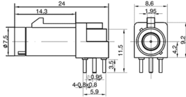
FAKRA SMB-R-M-RA-P-1
