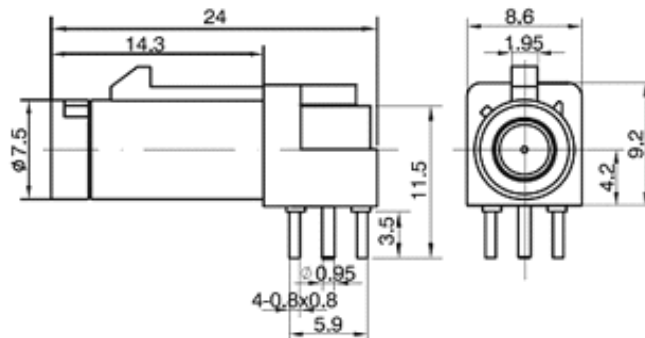
FAKRA SMB-R-M-RA-P-3
